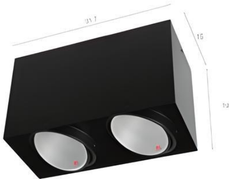
VL-3-TB-557-2 E27 (PAR30) x 2
